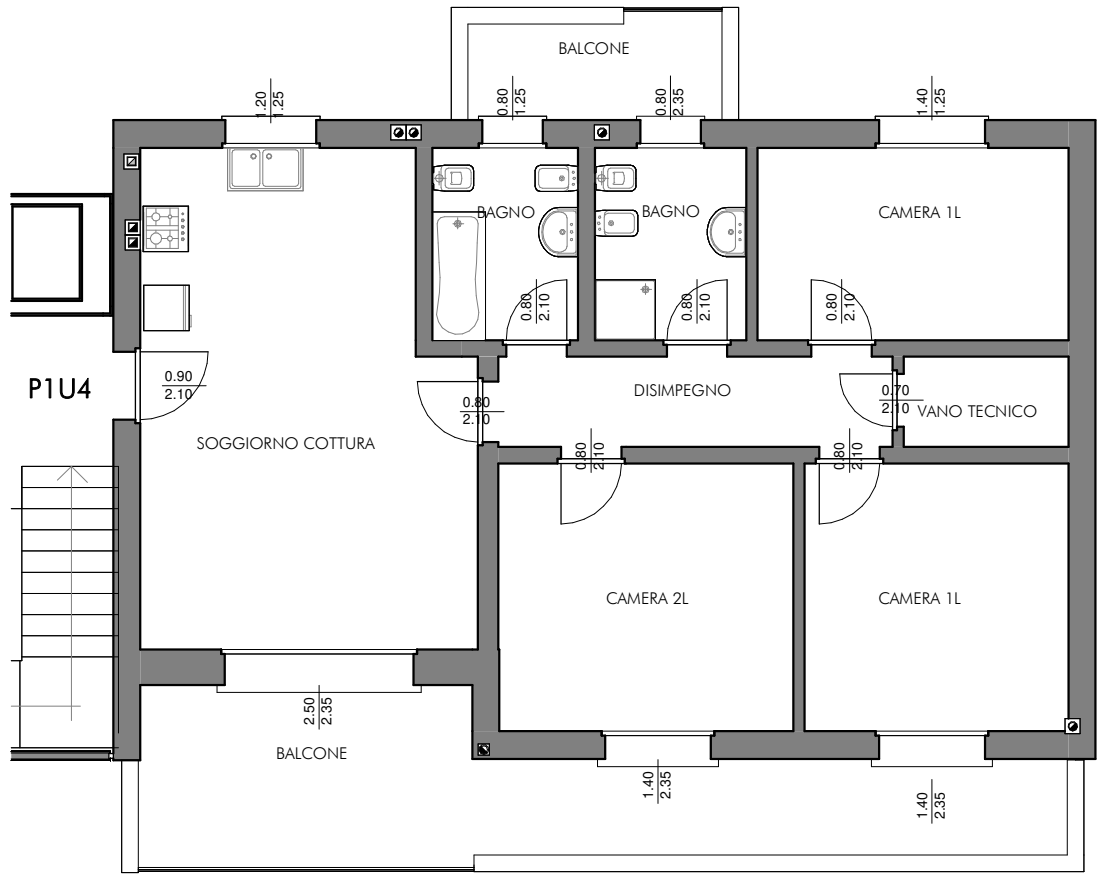
P1 UI4 - Pianta appartamento - piano primo 1:100
