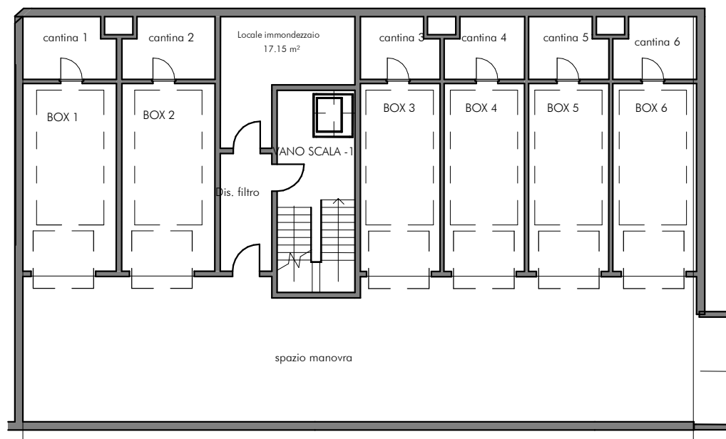
Pianta Piano interrato 1:200
