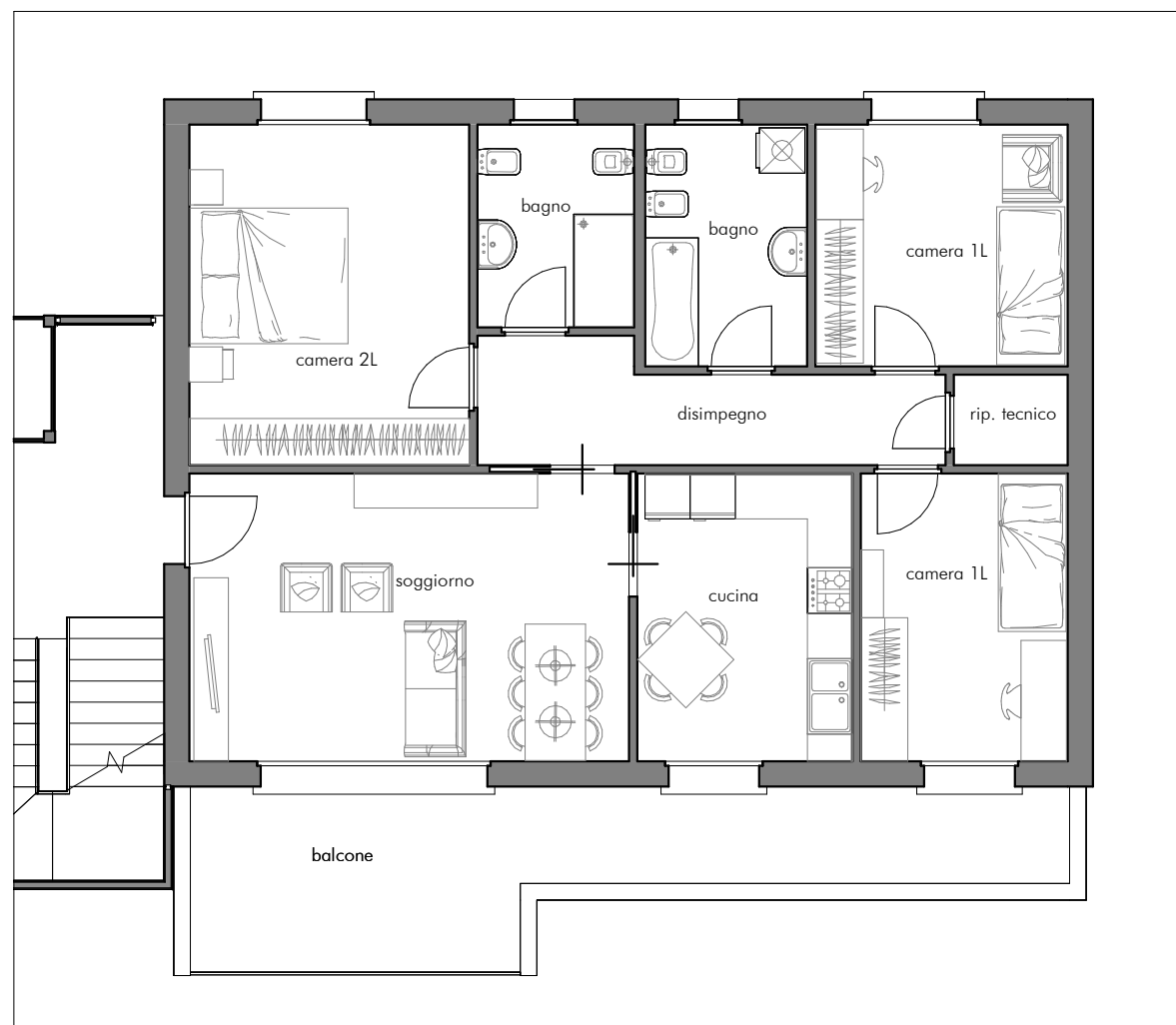
UI 5 Pianta piano primo 1:100
