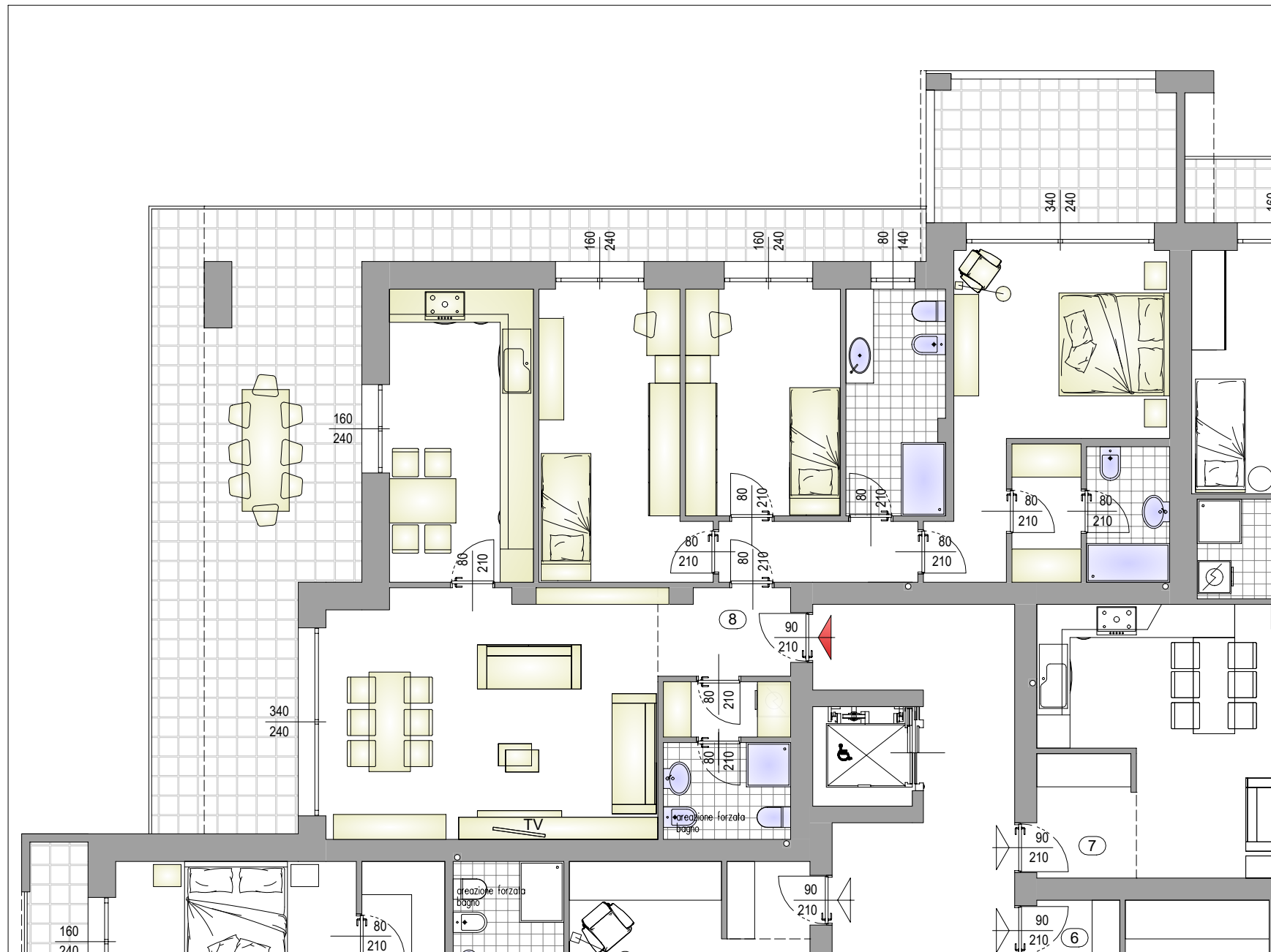
PIANO PRIMO APPARTAMENTO 8
