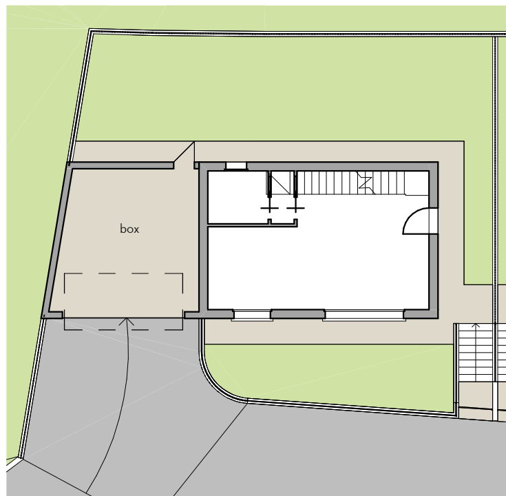
Piano terra generale 1:200
