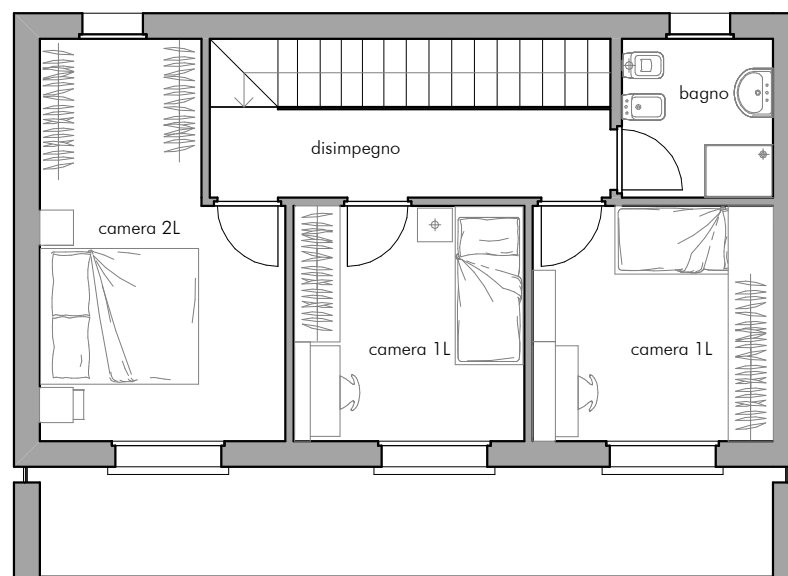
Piano primo 1:100
