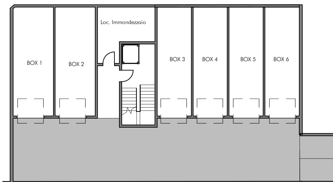
Pianta piano interrato 1:200
