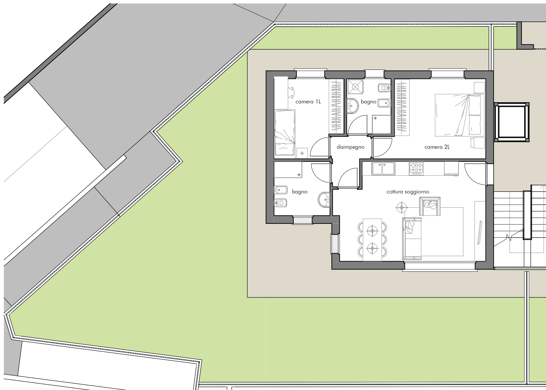
UI1 Pianta piano terra 1:100
