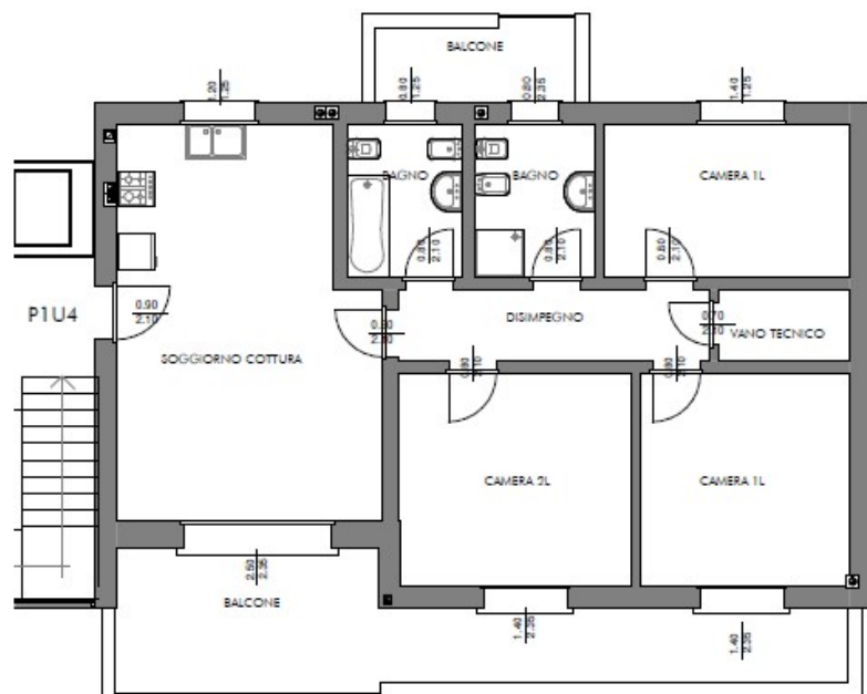
P1 U14 - Pianta appartamento - piano primo 1:100
