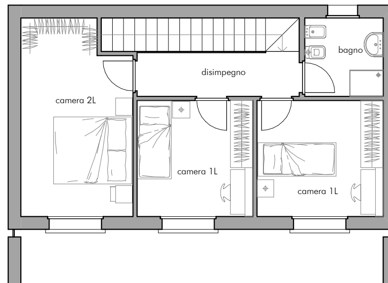
Piano primo 1:100
