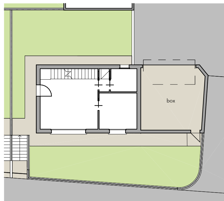
Piano terra generale 1:200
